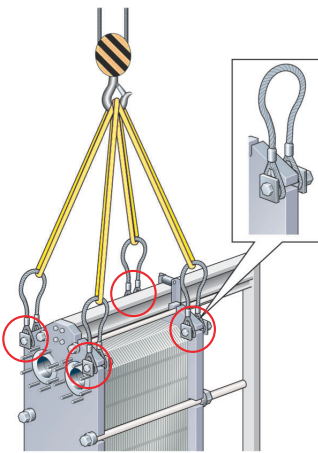
Kuva 6: Nostolaite malleille T25, MX25 ja MA30-S.
