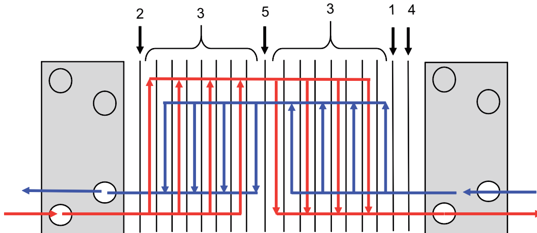
Kuva 4: Esimerkki monikiertoisesta kokoonpanosta
