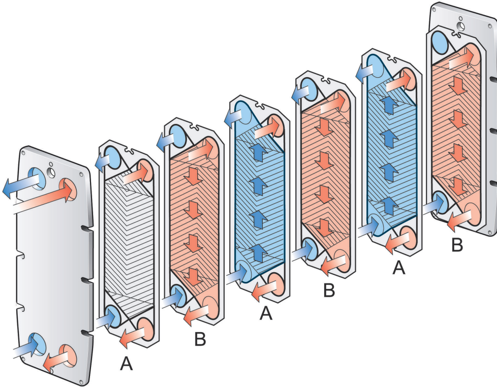
Kuva 2: Levypakka-asettelun periaate, tiivisteet runkolevyä kohden.
