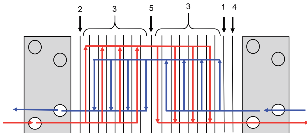
Kuva 3: Esimerkki monikiertoisesta kokoonpanosta
