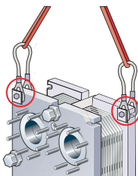
Kuva 8: Mallien AQ4T, AQ2T, AQ3 ja AQ2L nostaminen
