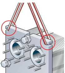
Kuva 5: Mallien AQ1, AQ2, AQ4, AQ1A, AQ2A, AQ2S ja AQ1L sekä mallien AQ3 ja AQ2L vanhojen versioiden nostaminen
