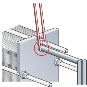
Kuva 6: Mallien AQ1, AQ2, AQ4, AQ1A, AQ2A ja AQ1L sekä mallien AQ3 ja AQ2L vanhojen versioiden nostaminen
