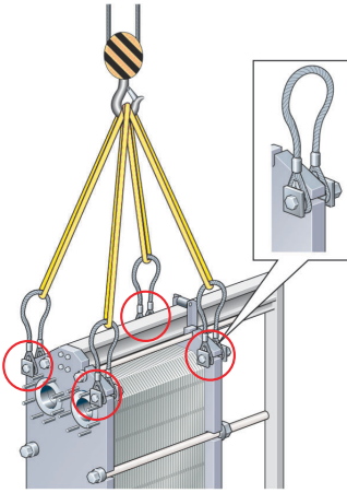
Kuva 6: Nostolaite malleille AQ10T ja AQ10.
