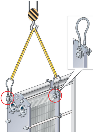
Kuva 5: Nostolaite malleille AQ6, AQ4L, AQ6L, AQ8 ja AQ8S.
