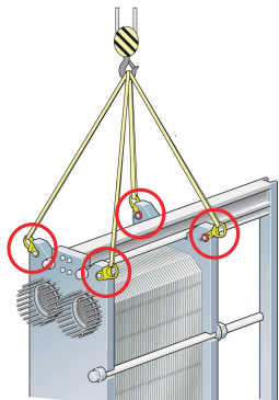
Kuva 7: Nostolaite malleille AQ18 ja AQ14L. Kiinnitysvälineitä ei vaadita.
