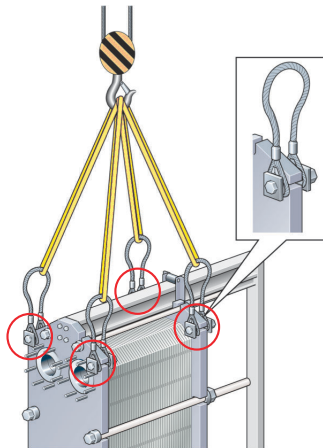
Kuva 6: Nostolaite malleille AQ14 ja AQ14S. Kiinnitysvälineitä on käytettävä.
