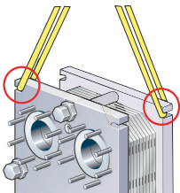
Kuva 4: Mallien AQ4T ja AQ2T nostaminen
